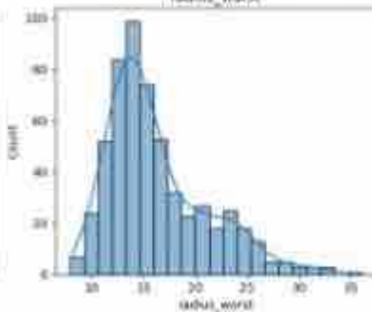
radius_worst
