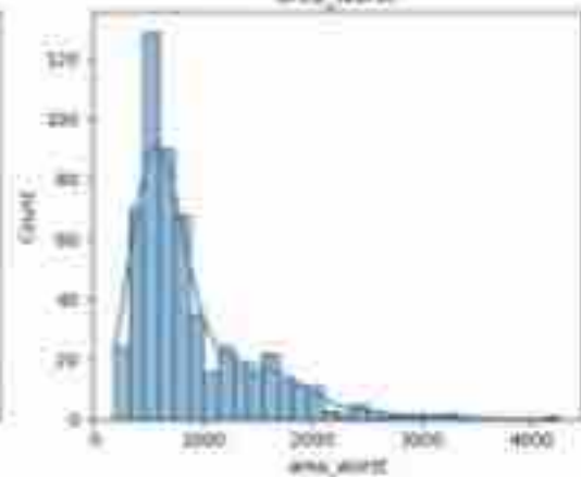
area_worst
